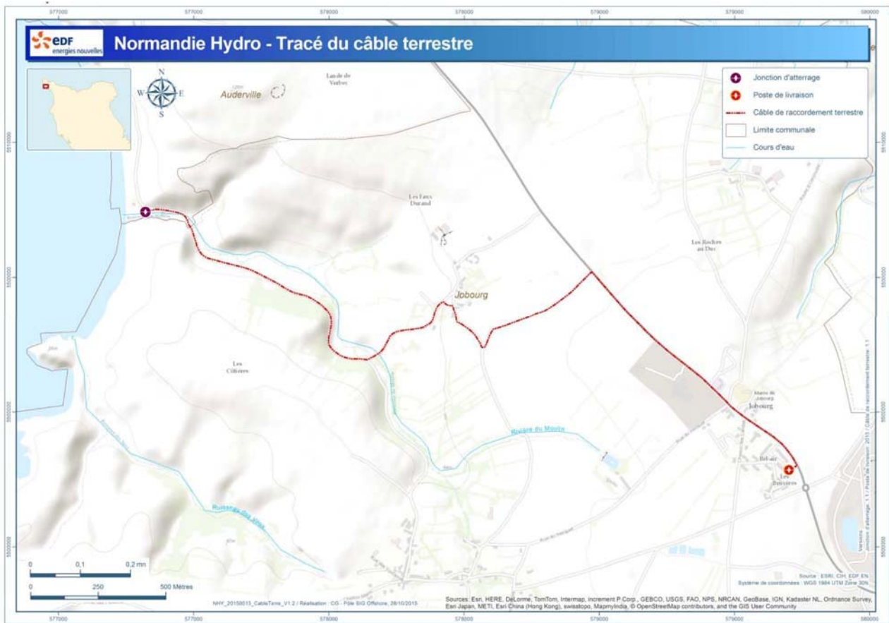
Figure 5 : tracé du câble de raccordement électrique terrestre depuis la jonction d'atterrage jusqu'au poste de livraison électrique (source : Etude d'impact)
