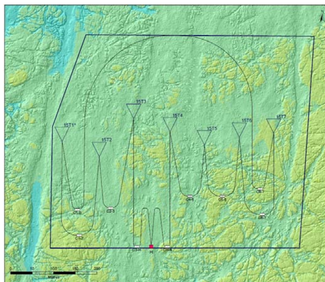
Figure 3 : Implantation des turbines, du hub de connexion sous-marin, des câbles et connecteurs électriques inter-hydroliennes sur la zone projet du projet Normandie Hydro (source : Etude d'impact)
