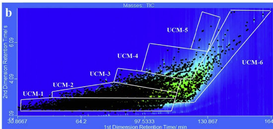
Figure 3: Chromatogramme d’une fraction aromatique du pétrole “Well CI 20-138” obtenu par GCxGC/TOF-MS (Weng et al. 2015).
