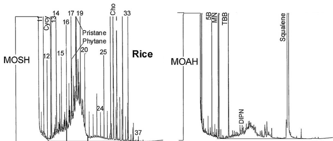
Figure 1: Exemple de chromatogrammes obtenus par GC/FID lors de l'analyse d'un échantillon de riz emballé dans un emballage en papier et carton imprimé (Biedermann and Grob 2012a).
